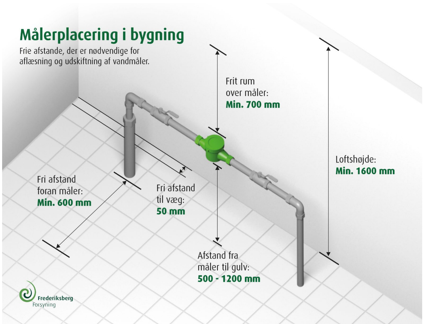
Illustration 2: Målerplacering i bygning
